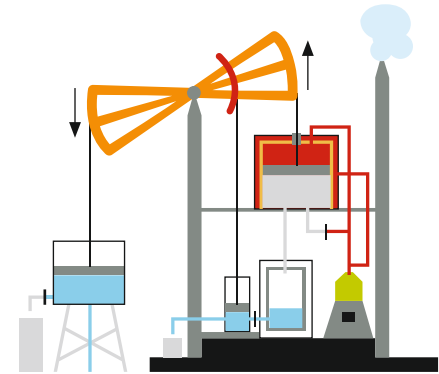
Newcomenův atmosférický parní stroj – přítel horníků
