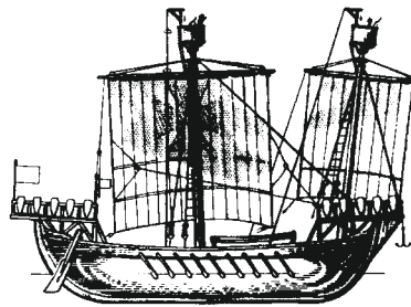
Normandská loď
