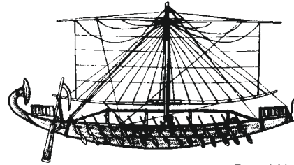
Egyptská loď
